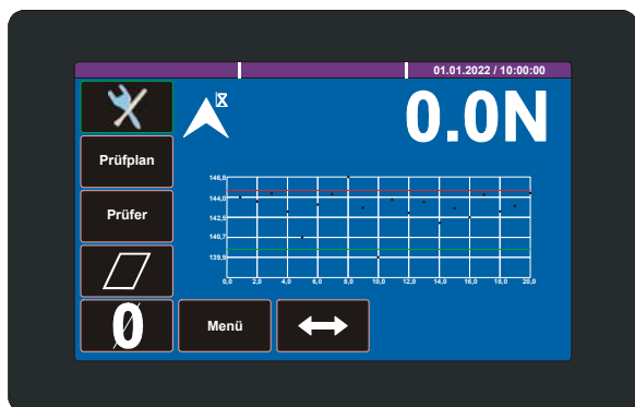
FMS mit grafischer Darstellung von gemessenen Spritzenwerten
