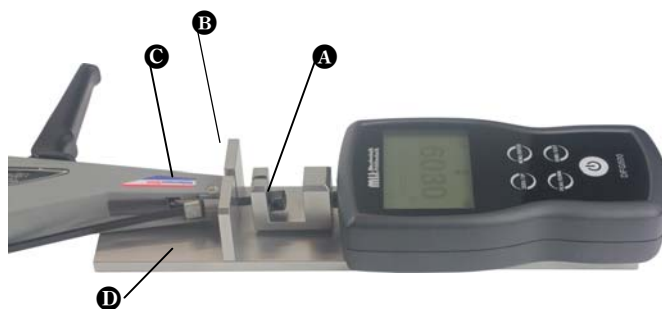
Prüfaufbau mit DFG-KBP 500V
