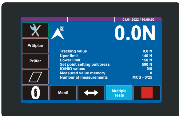
FMS mit optionaler MFU Firmware-Erweiterung
